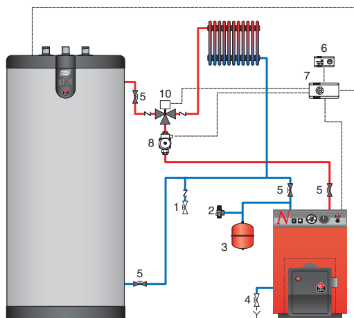
Схема с трехходовым клапаном с приводом.
